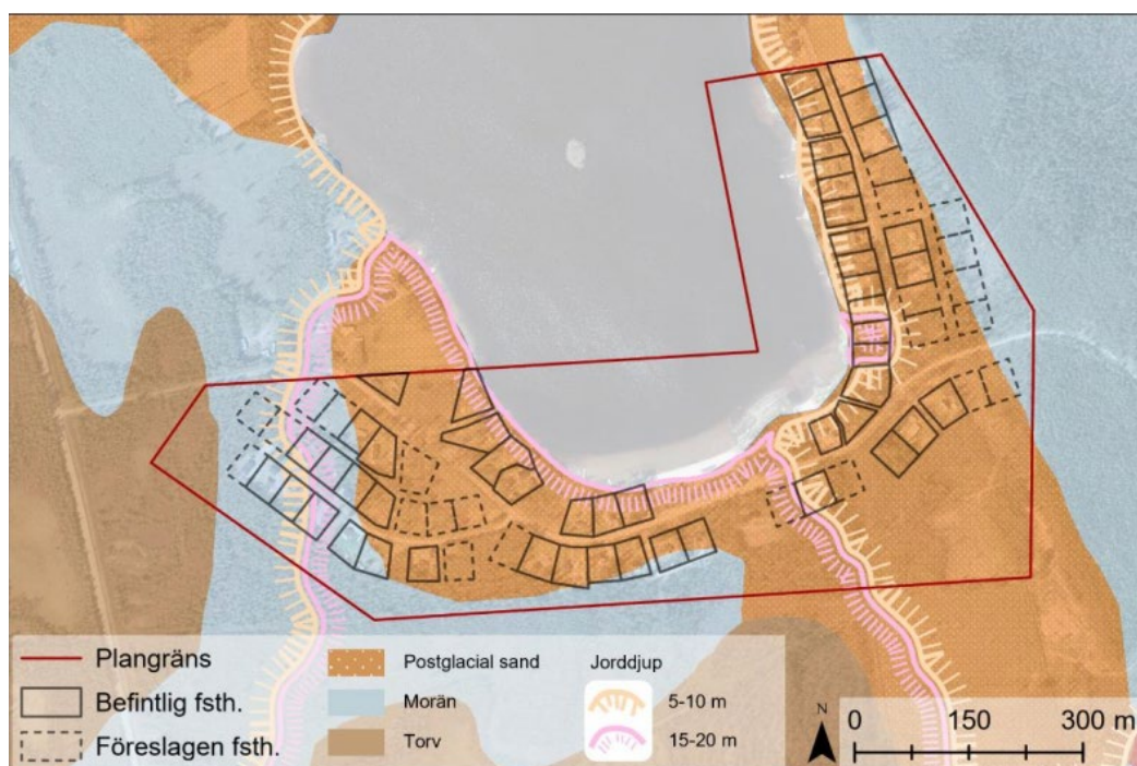
Jordarterna och jorddjupens utbredning. Observera att föreslagen fastighetsplacering (streckad linje) och plangräns (röd linje) har justerats sedan underlaget i figuren togs fram.
