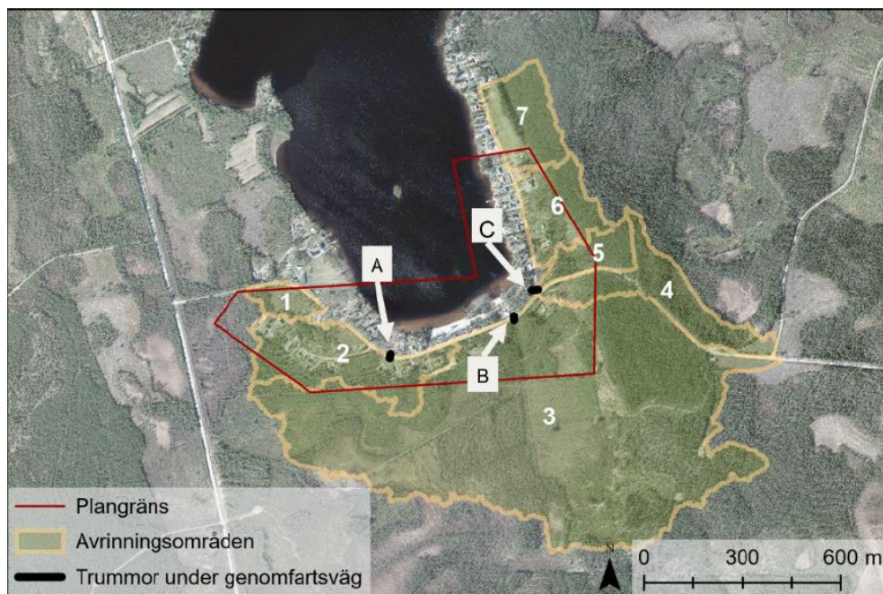
Avrinningsområden som bidrar med avrinning inom planområdet. Observera att plangräns (röd linje) har justerats sedan underlaget i figuren togs fram (Tyréns)
