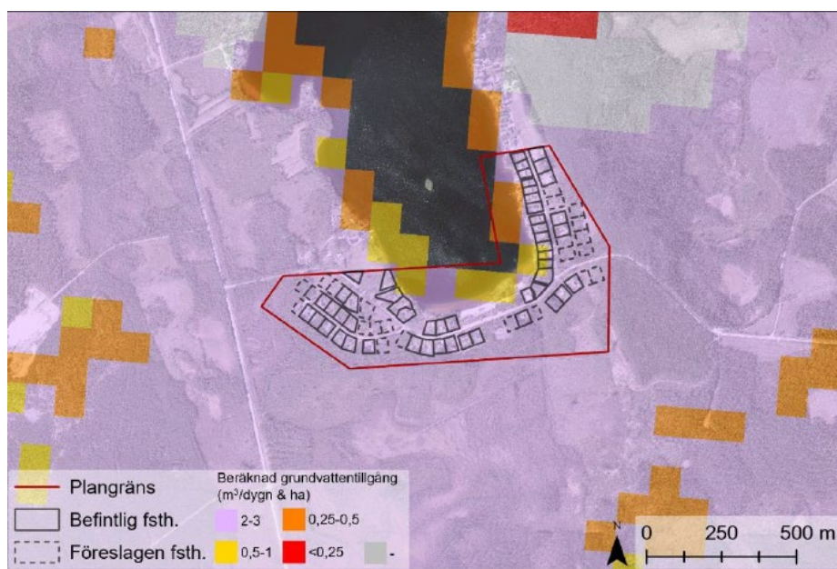
Beräknad grundvattentillgång i små magasin. Observera att föreslagen fastighetsplacering (streckad linje) och plangräns (röd linje) har justerats sedan underlaget i figuren togs fram. (Tyréns).
