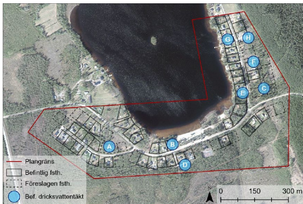
Befintliga kända dricksvattentäkter i området, (Tyréns).
