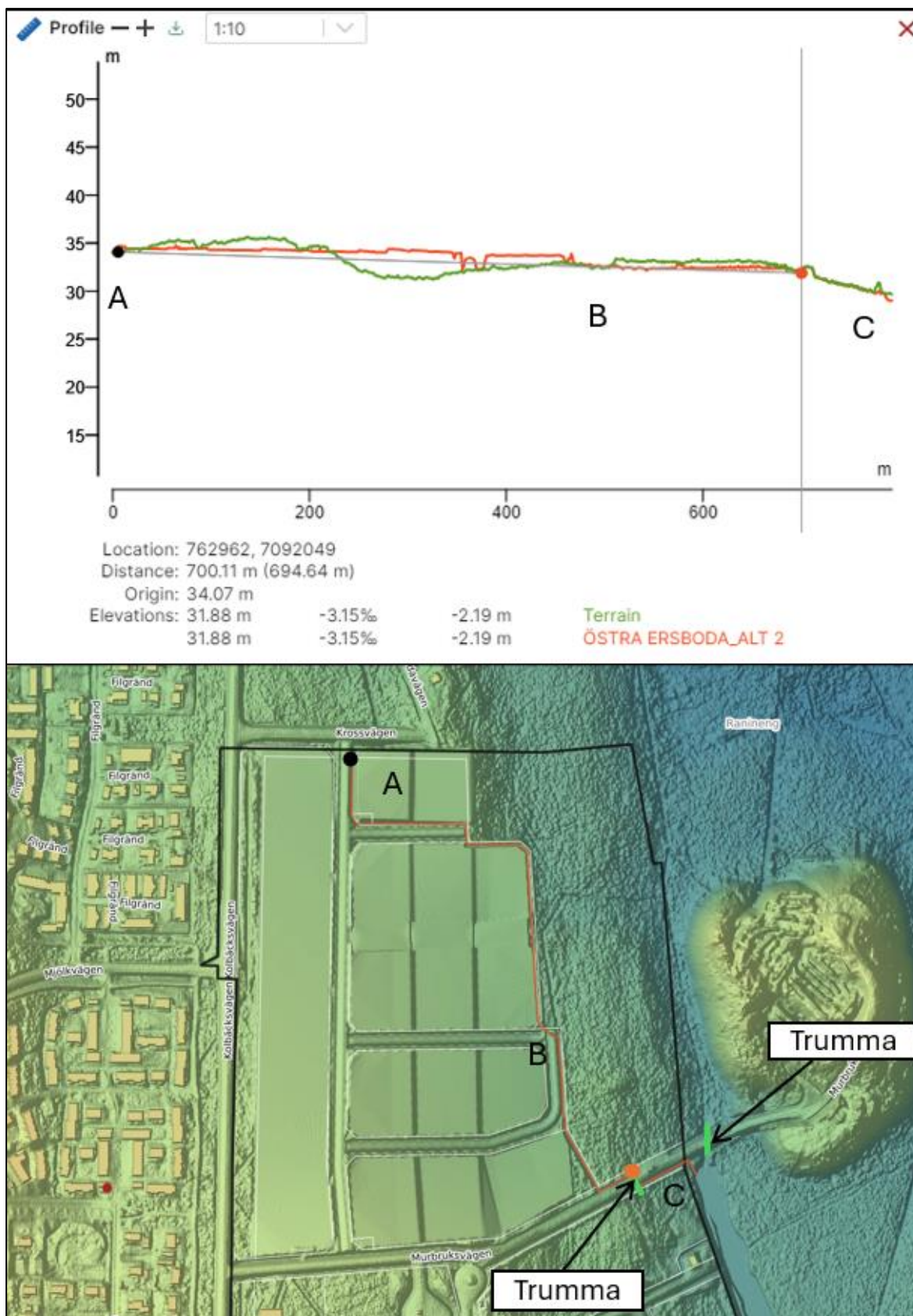
Figur 39. Profil över föreslaget dike till dagvattendamm (Scalgo Live, 2024). Föreslagen dikesbotten och höjdsättning (Sigma, 2022) visas med grönt i profil och befintliga höjder i orange. Profilens utbredning går från norr till söder (riktning: vänster-höger). Markering A-C är referenspunkter.
