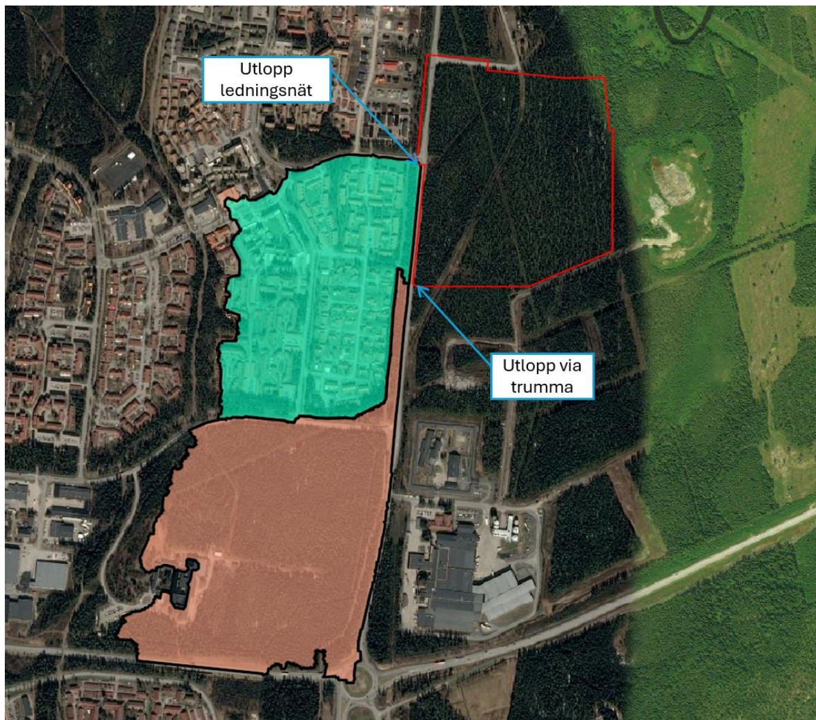
Figur 9. Avrinningsområdena uppströms, som avrinner in mot utredningsområdet (Scalgo Live, 2024). Utredningsområdet visas i rött.
