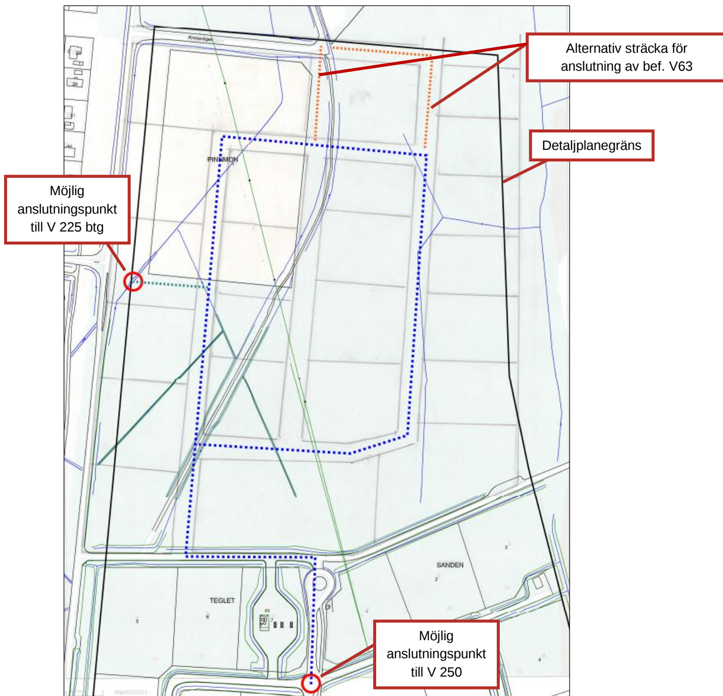
Figur 46. Schematisk ledningsdragnig för dricksvattenledningar inom utredningsområdet. Utkast på plankarta enligt tidigare förslag.
