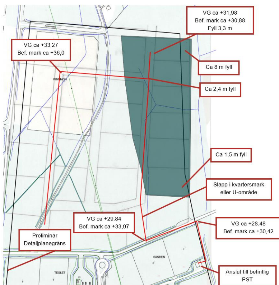
Figur 48 för ungefärligt område som kräver fyll. För att kvartersmarken öster om gatan ska hamna i samma nivå som gatumark krävs upp till ca 8 m fyll. Observera att mängden fyll är beroende av höjdsättningen inom hela området. Föreslagen ledningsdragning kräver släpp i kvartersmark eller u-område längst i söder. Det här alternativet påverkar även placeringen av diken för avledning av dagvatten mellan planerade fastigheter och det östra befintliga diket. Placeringen av dessa diken anpassas till lågpunkterna.
