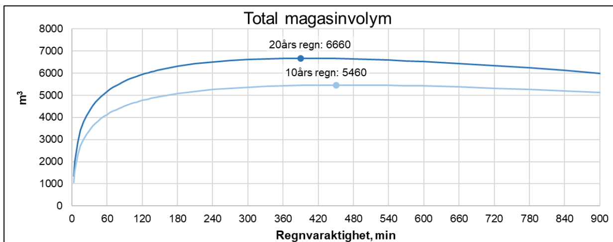
Figur 34. Erfordrad fördröjningsvolym för utredningsområdet, för fördröjning av ett regn med återkomsttiden 10 och 20 år.
