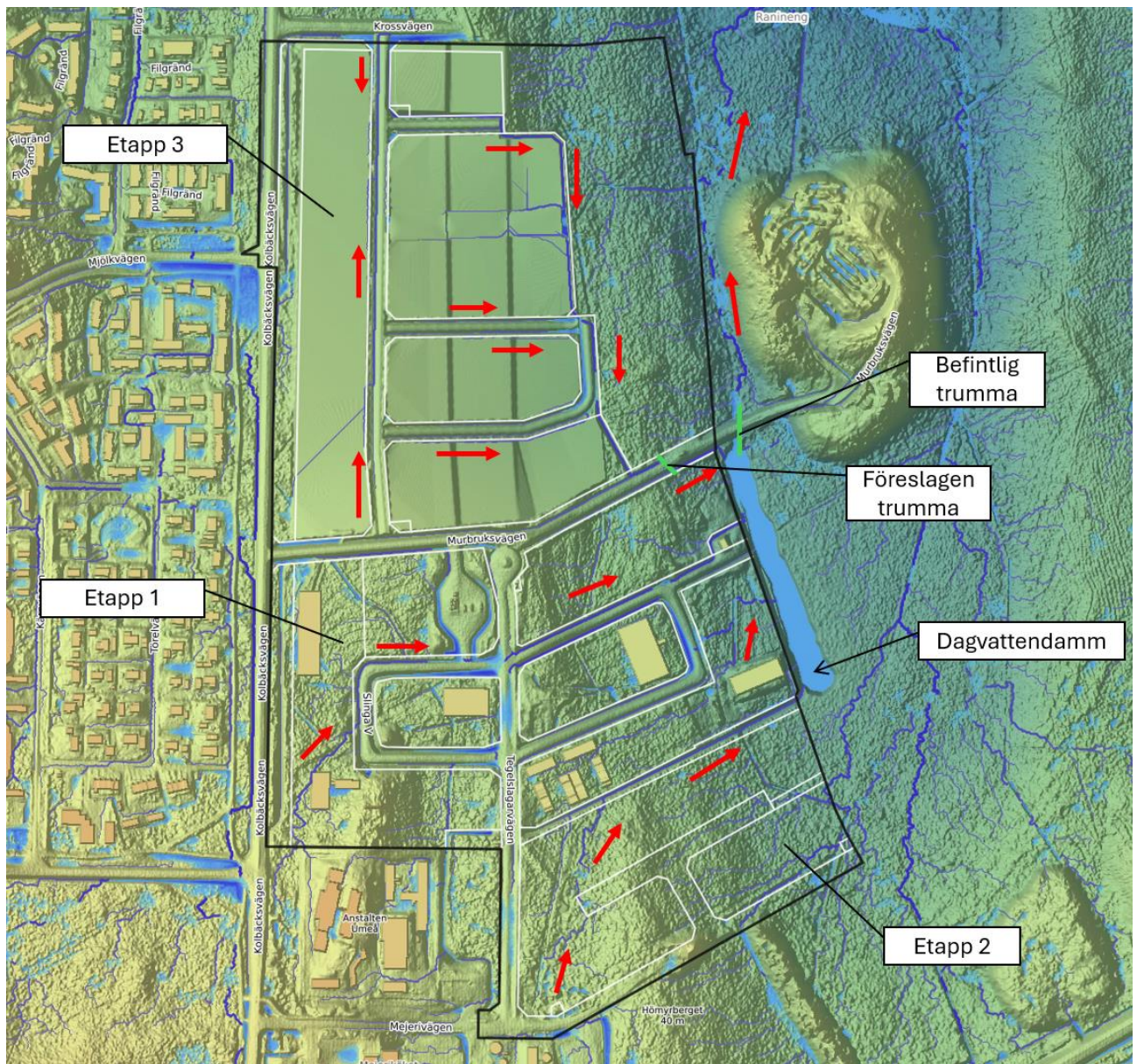
Figur 37. Schematisk skiss över föreslagen systemlösning, baserad på tidigare föreslagen höjdsättning Sigma (2022). Avledningen av dagvattnet sker via öppna dikesstråk mot sydöst, till föreslagen dagvattendamm (Scalco Live, 2024).
