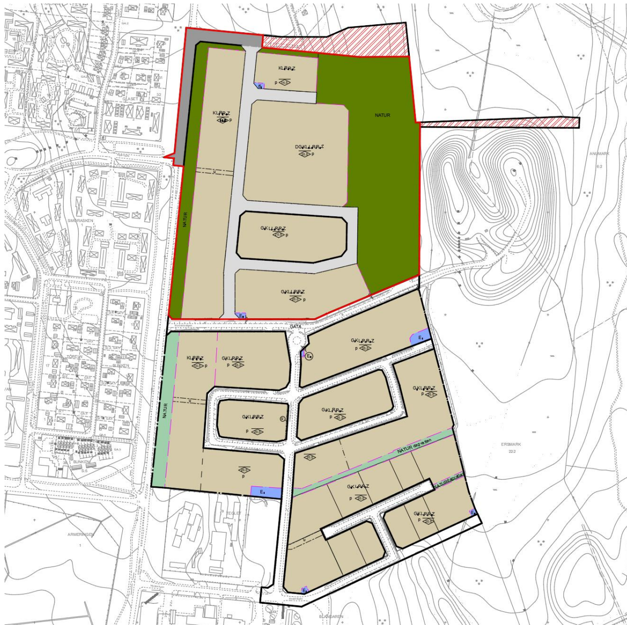
Figur 33. Planerad exploatering efter samrådshandling (Umeå kommun, 2024). Utredningsområdesgräns visas med röd linje. Rödskrafferade områden visar ytor som utgått ur detaljplanen.
