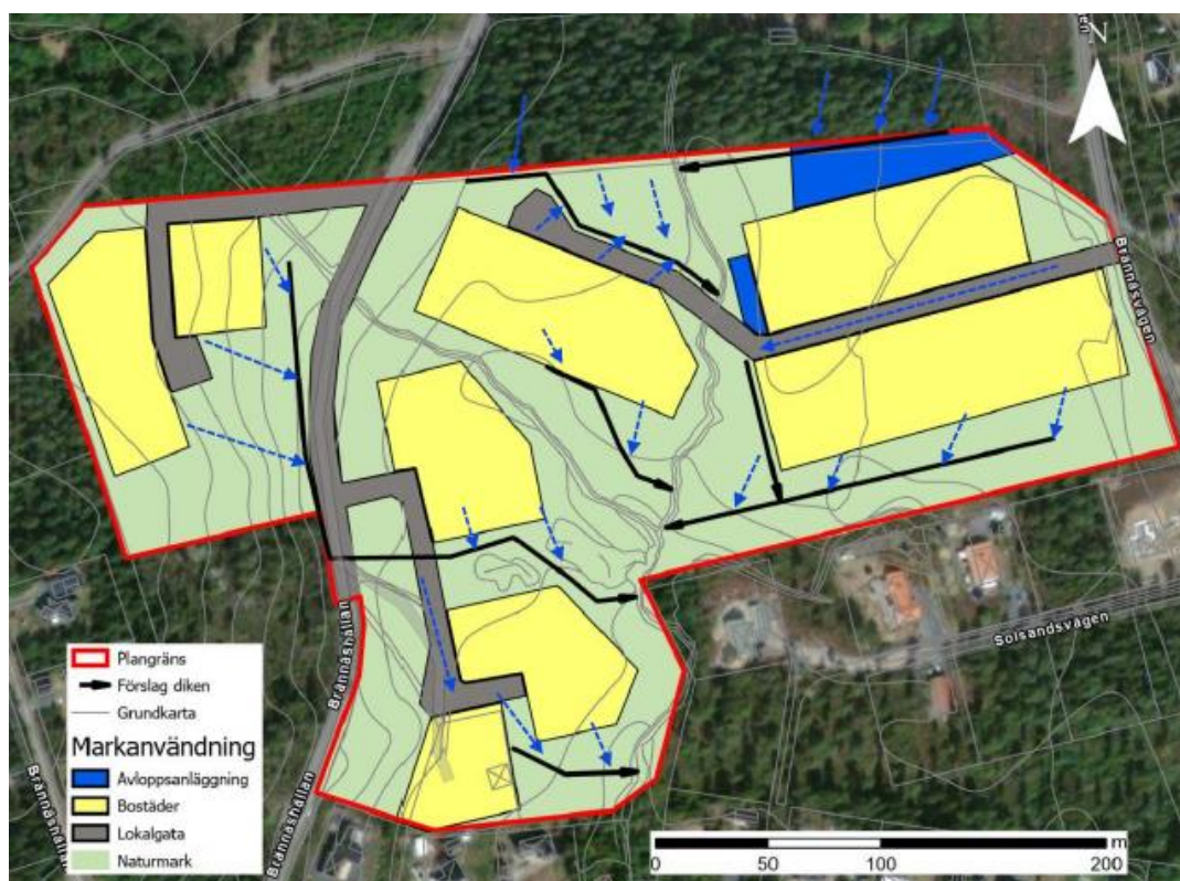
Figur 12. Förslag på placering av diken för fördröjning av dagvatten. Svarta pilar visar dikenens föreslagna placering och rinnvägar. Blå streckade pilar visar avrinning till diken.
