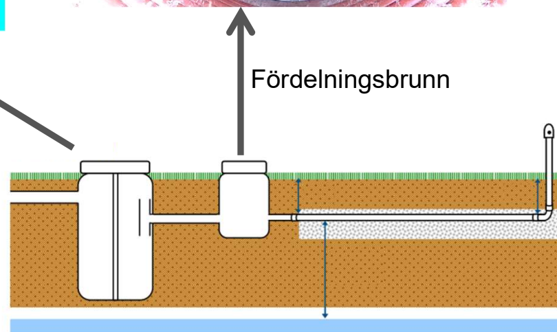
Slamavskiljare
