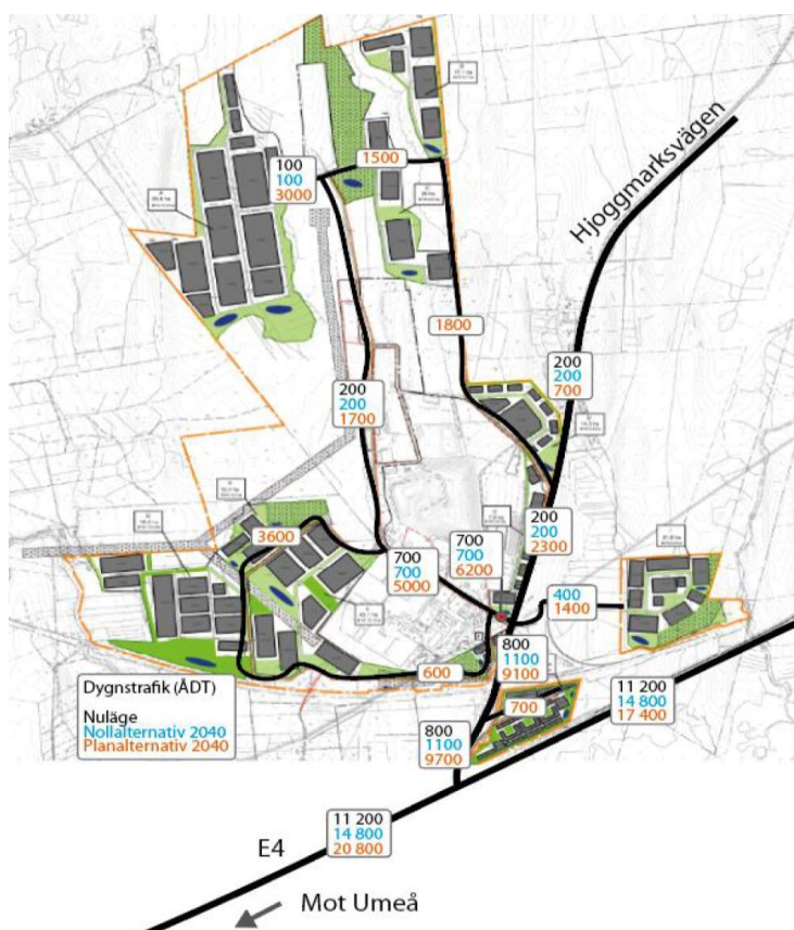
Figur 1. Nätutläggning av trafik, detaljplan Nyskogen 1:1
